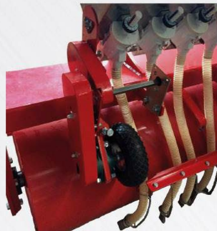
Particolare trasmissione meccanica
